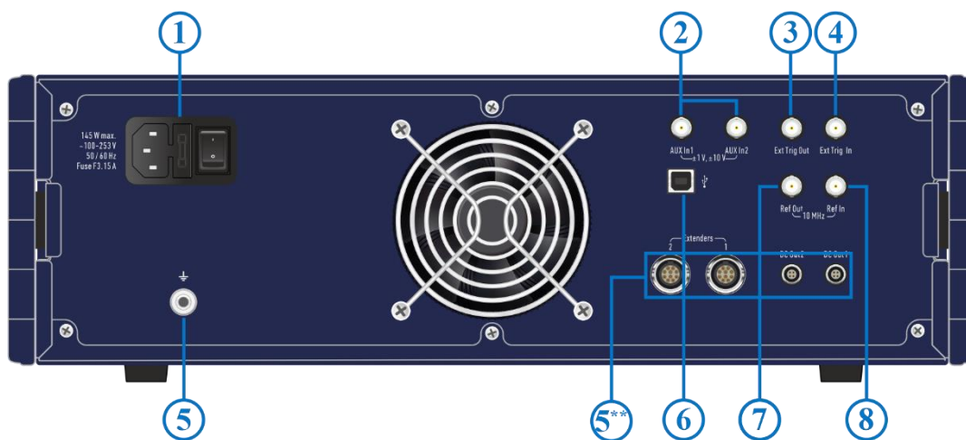
Рисунок 4.28 Задняя панель
