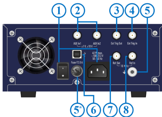
Рисунок 4.6 Задняя панель
