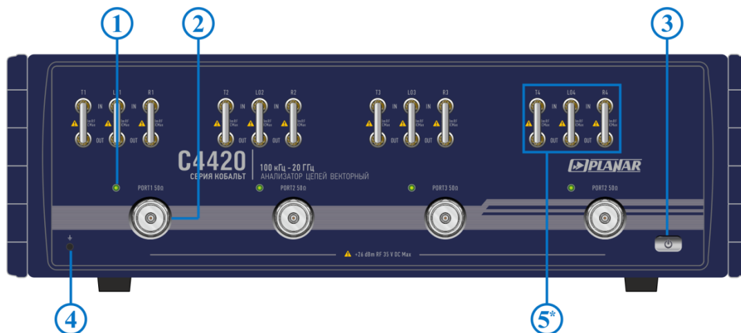
Рисунок 4.29 Передняя панель
