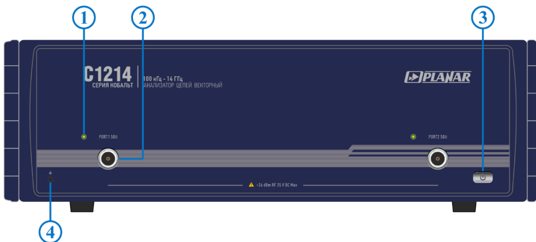
Рисунок 4.7 Передняя панель
