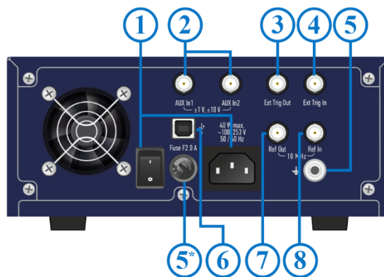
Рисунок 4.4 Задняя панель
