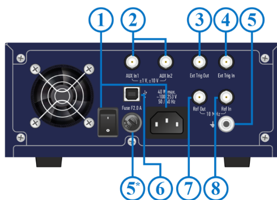
Рисунок 4.2 Задняя панель
