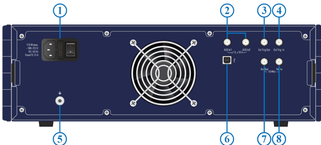
Рисунок 4.10 Задняя панель
